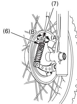
(6) Lukkomutteri (A) Vähentää vapaaliikettä (7) Säätömutteri (B) Lisää vapaaliikettä
